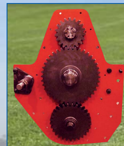
Engranajes laterales Transmission latérale Side drive gears
