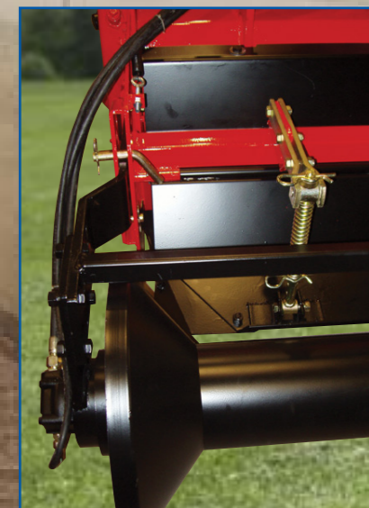
Cono desplazable Cone deportable Adjustable roller cone
